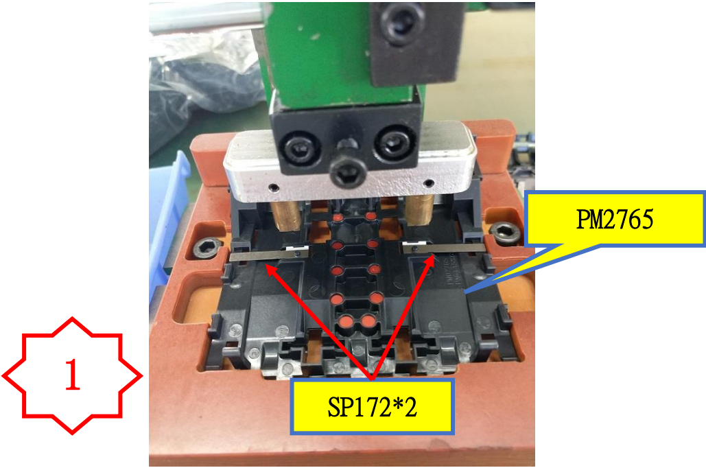
图一，将 PM2765 放入治具上，在 PM2765 两边的柱子上放入 SP172，方向如上图所示，然后进行压合
