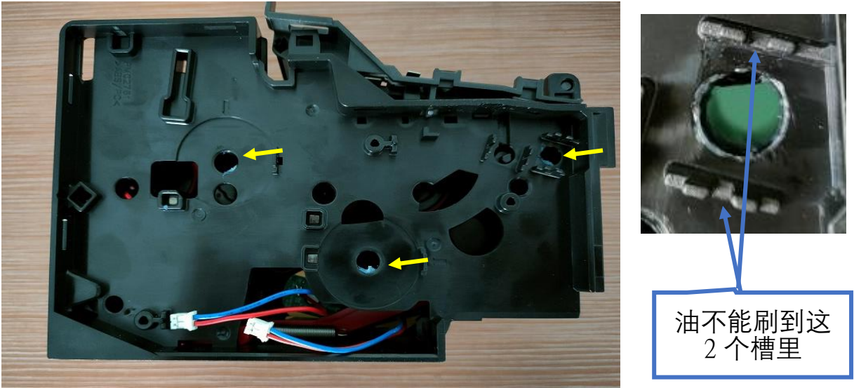
图一，用点油机在黄色箭头的孔各加 0.0071g NYE368F 油
