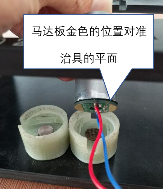
图一, 将两个马达组件装到治具上, 注意方向
