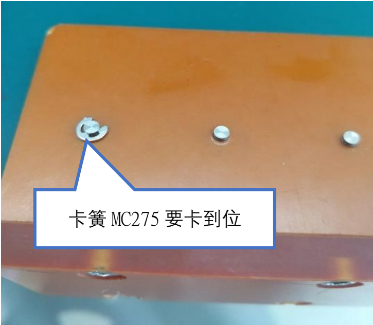
图二，在轴 MC2339 上卡入卡簧 MC275
