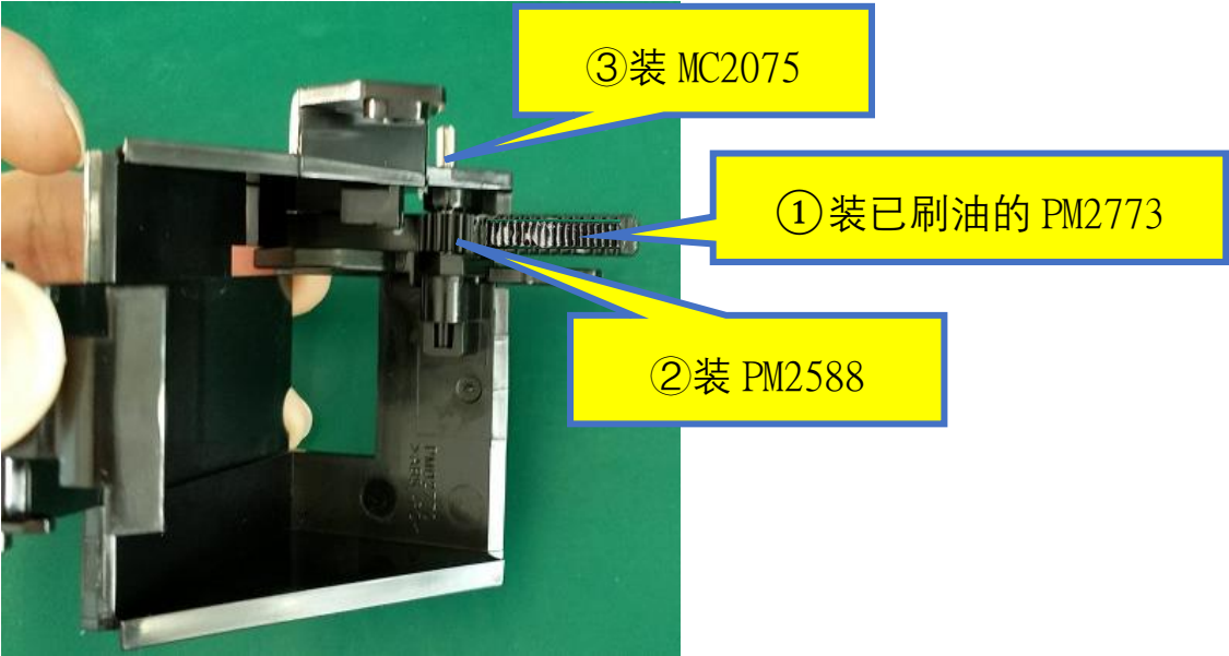
图一, ①将已刷油的 PM2773 装到 PM2770 里, ②将 PM2588 放到位, ③穿入一个 MC2075。
