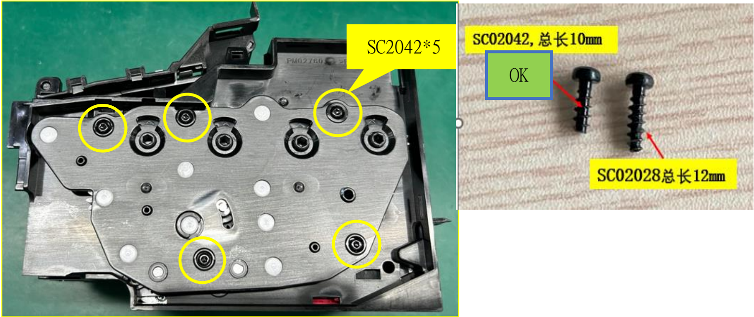
图二，在 PM2768 图示位置上打入五颗 SC2042 螺丝，注意装配到位后不能有滑牙或打不到位问题。
