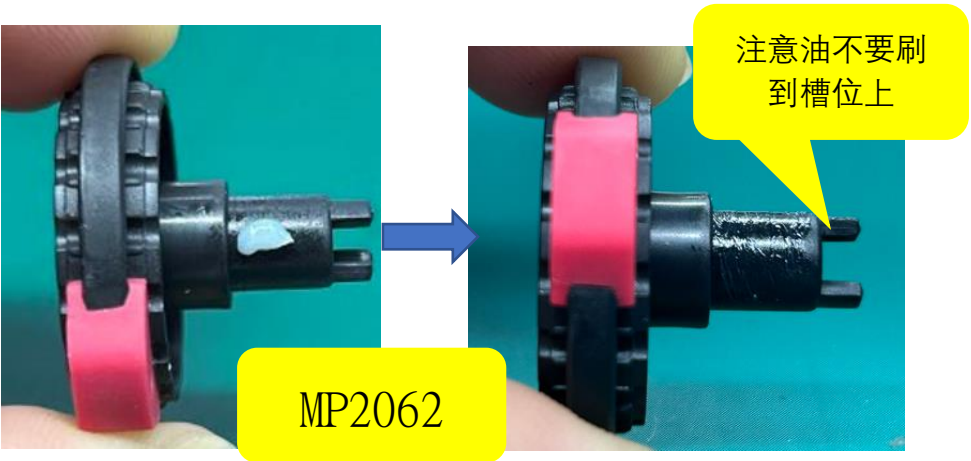
图一，用点油机在 MP2062 加大约 0.0071g NYE368 油，然后用毛刷将油均匀刷在柱子上。
