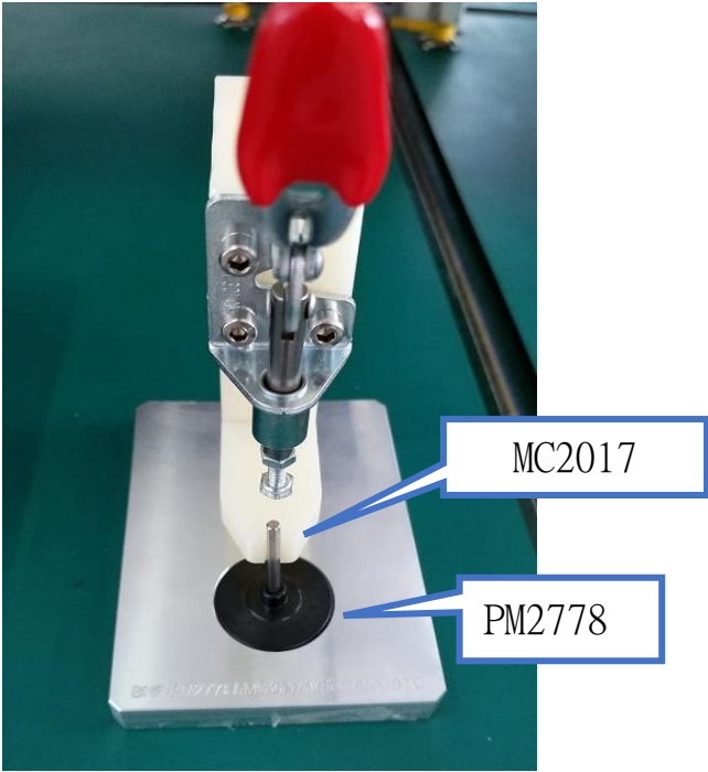
图一，在 PM2778 上压入一个 MC2017
