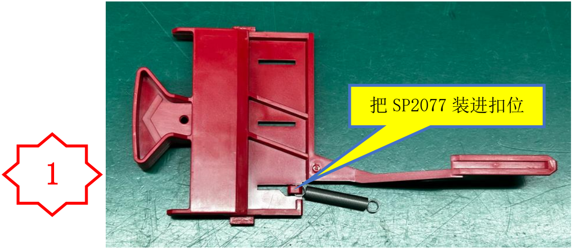
图一, 将 SP2077 弹簧扣入已刷油的 PM2767 卡扣里面
