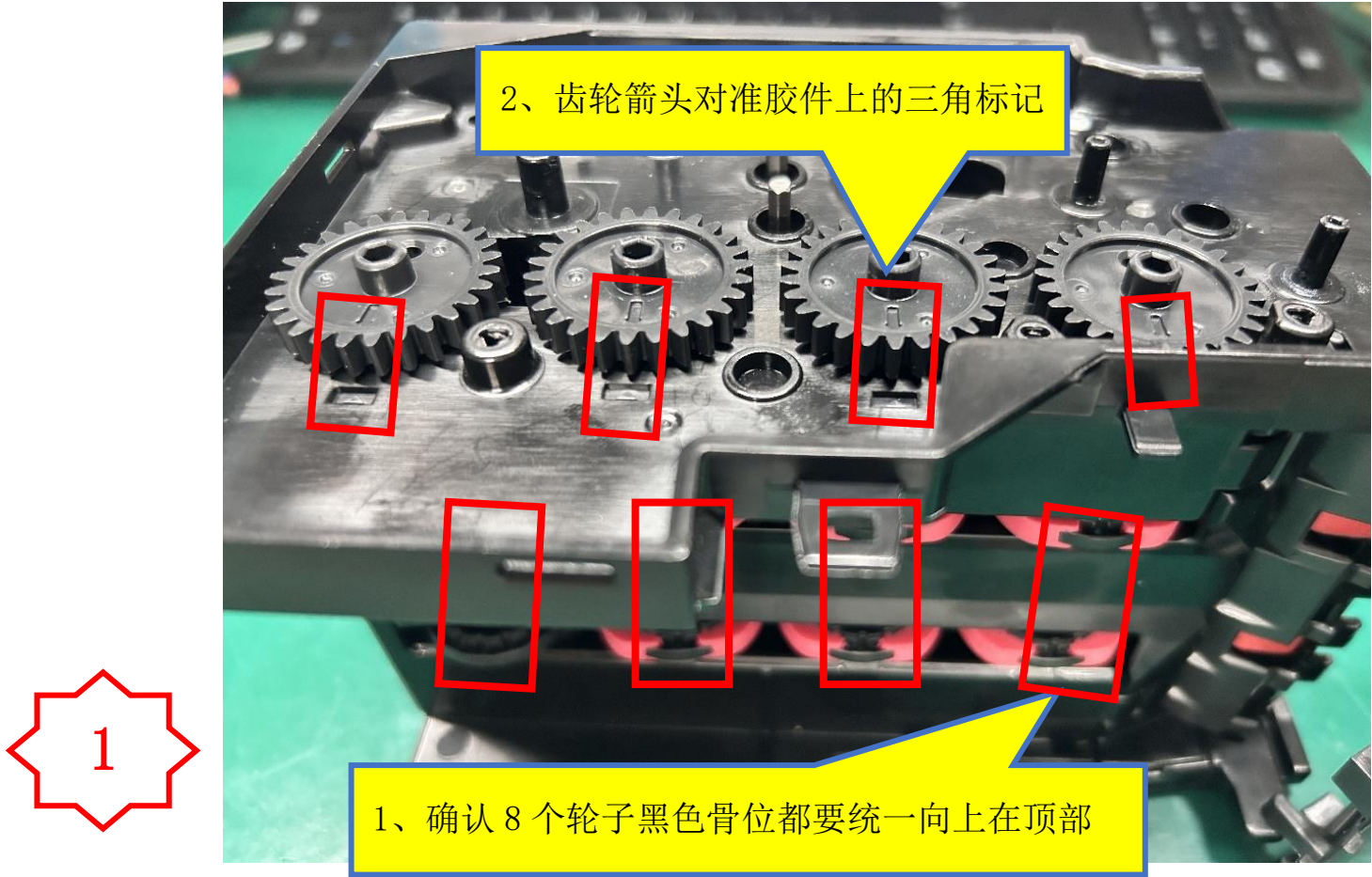
图一, 在 PA3122-3 上图示的 4 个孔分别装上 PM2776, 装入时请注意 PA3128 上的 8 个轮子统一方向, 黑色骨在顶部居中, 再将齿轮箭头对准胶件上的三角标记。
