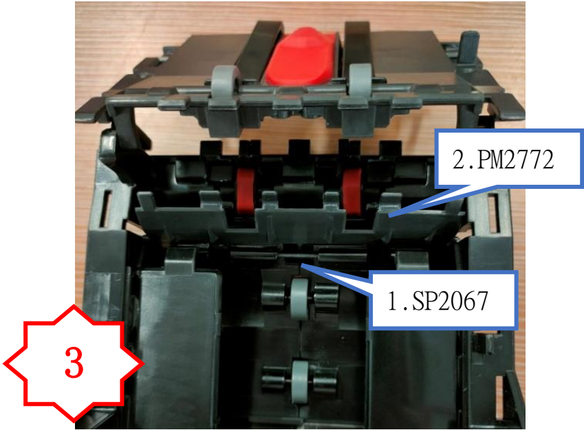
图三，将 SP2067 装到孔里, 然后装入 PM2772 到槽里
