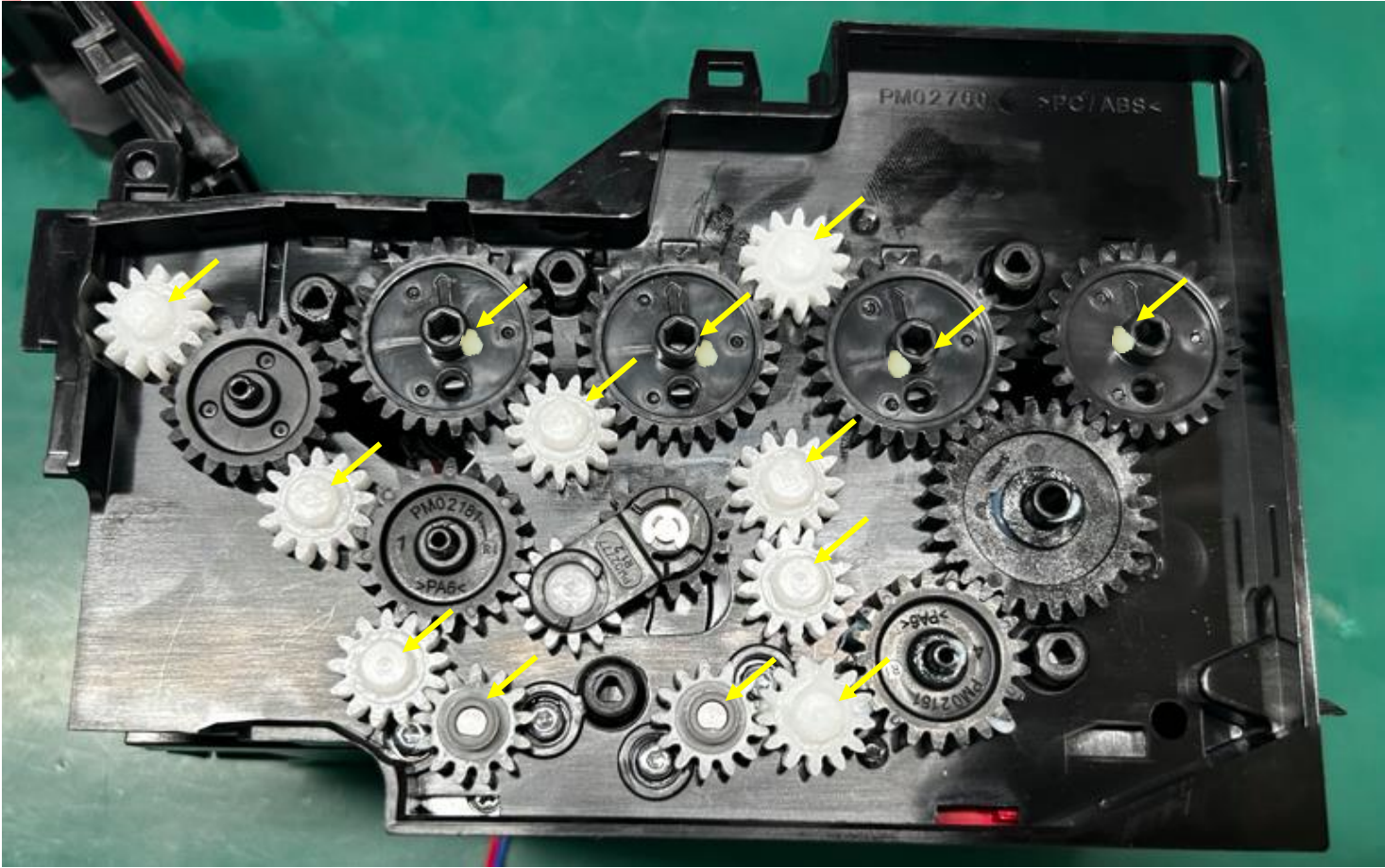
图一，黄色箭头标示位置柱子侧面点上适量的油脂（共 14 处）。
