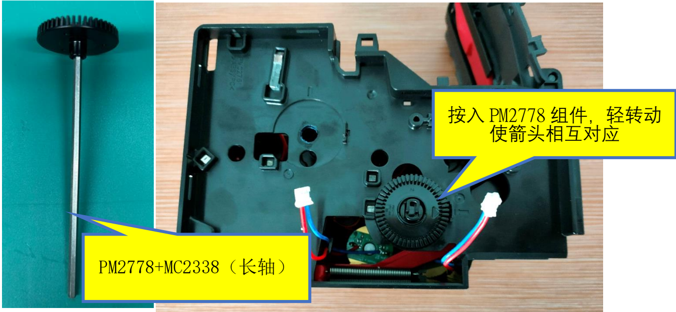
图二，装入一个 PM2778+MC2338 (长轴)，压到位后，PM2778 上的箭头和组件上的箭头对应。
