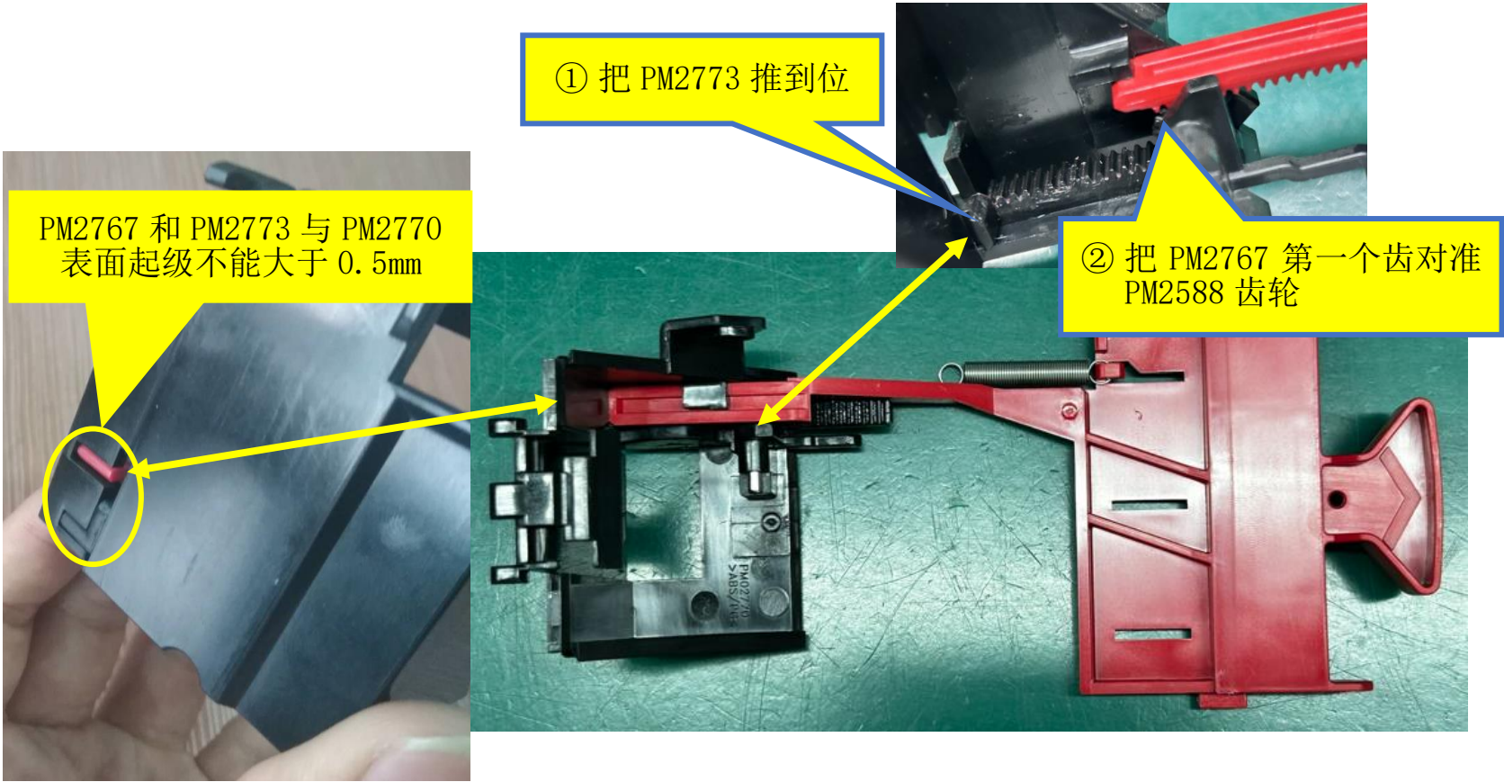
图二, ① 把 PM2773 推到位, ② 把 PM2767 第一个齿对准 PM2588 齿轮, 检查 PM2767 和 PM2773 与 PM2770 表面起级不能大于 0.5mm
