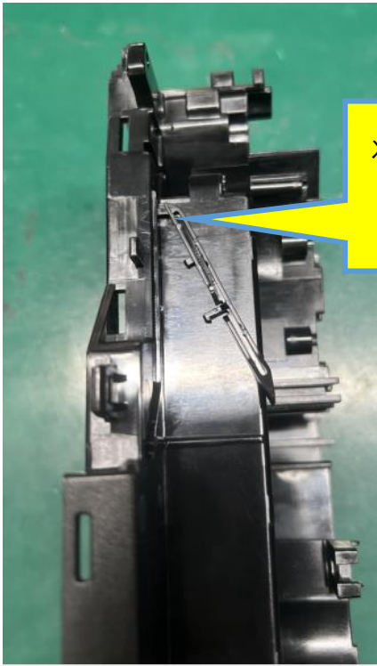
图二，将 PM2971 头部扣位先装入 PM2760 平面上的第一个孔中，再将后面的扣位推入后面的孔，确认卡扣装配到位。
