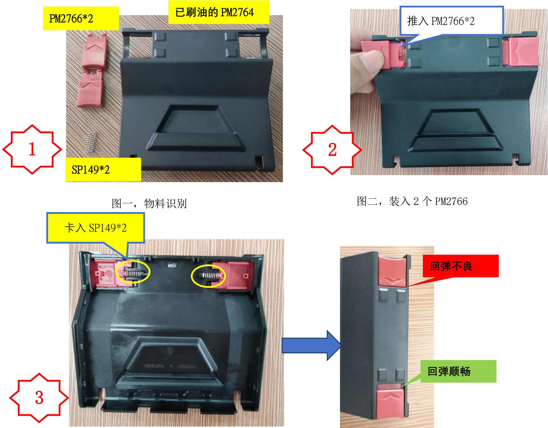
图三, 卡入 2 个 SP149, 检查 2 个 PM2766 是否可回弹复位
