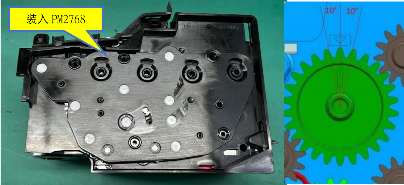
图一，注意不可改变轮子的方向，装入 PM2768 齿轮盖，PM2776 的箭头和上方的箭头对齐偏差左右不可超过 10 度
