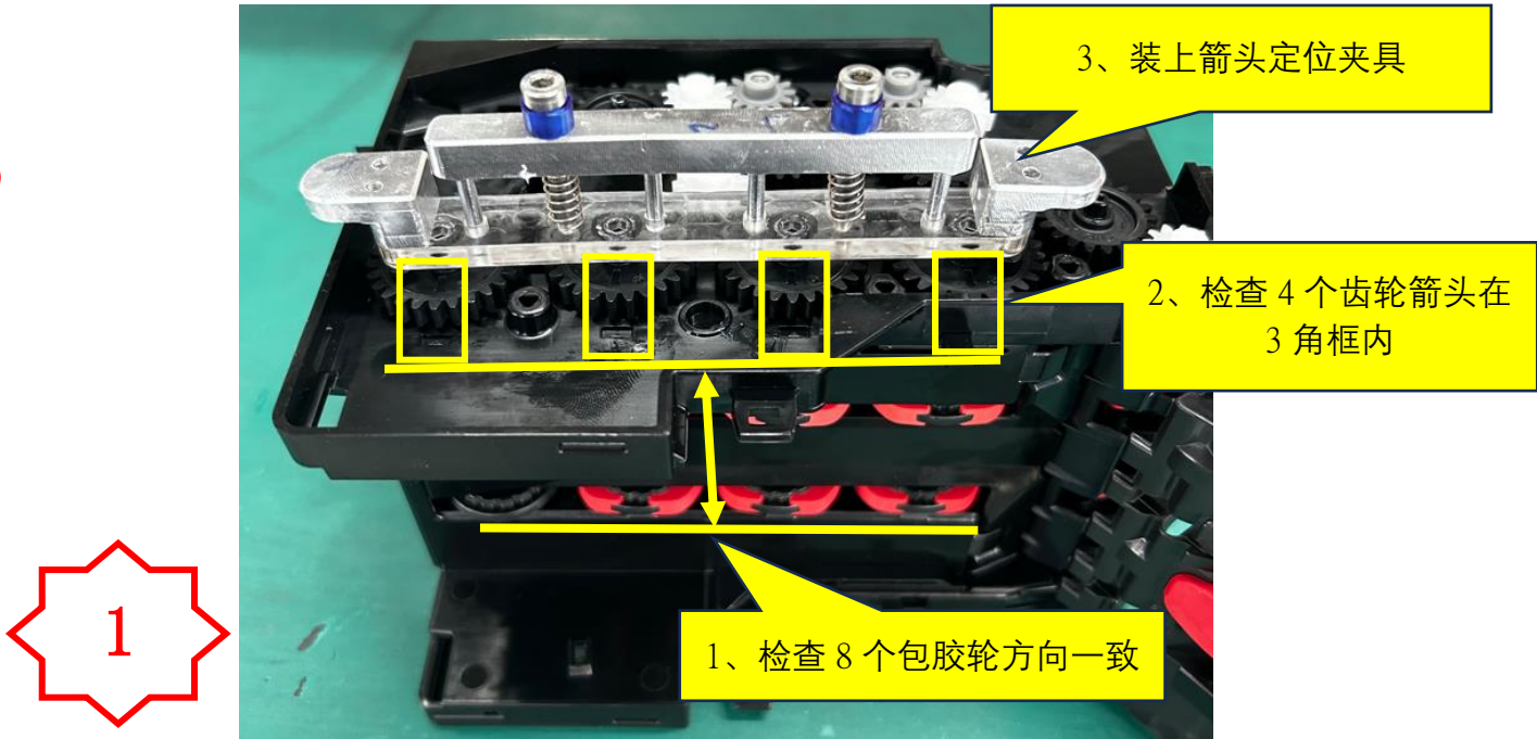
图一，检查 8 个包胶轮方向一致，4 个齿轮箭头在 3 角框内，再装上箭头定位夹具。
