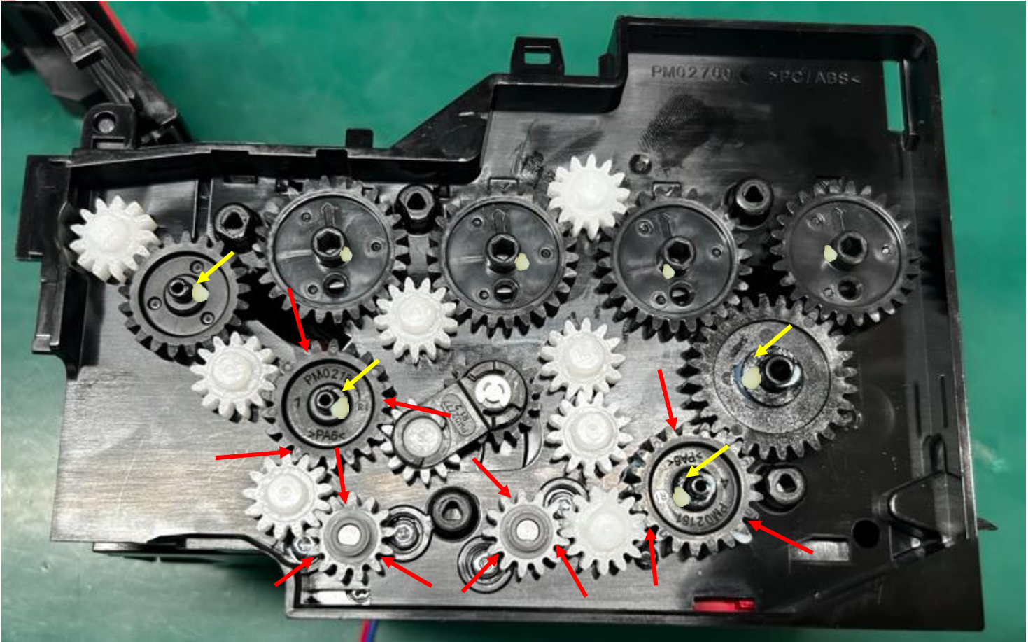
图一，黄色箭头在齿轮平面上的骨位点上适量的油脂（4 处），红色箭头点在齿轮齿上（12 处），总共 16 处。
