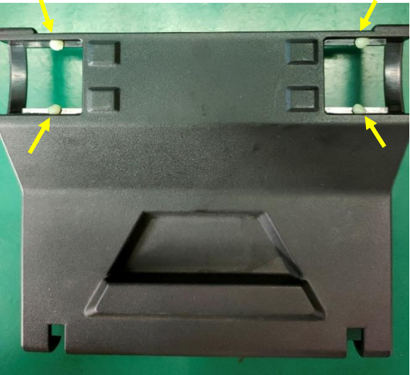
图一, 用点油机在 PM2764 的 4 处滑槽各加大约 0.0071gNYE 368F 油
