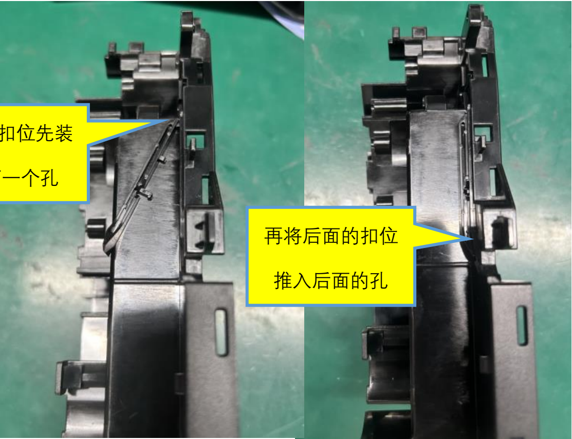
图二，将 PM2970 头部扣位先装入 PA3125-1 上的 PM2761 平面上的第一个孔中，再将后面的扣位推入后面的孔，确认卡扣装配到位。
