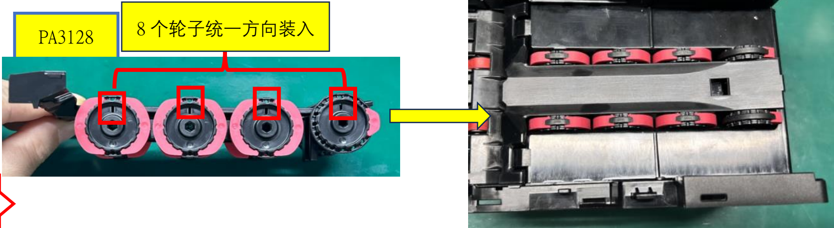
图一，检查 PA3128 组件 8 个轮子统一方向，然后将方孔对准导光柱装入 PA3123-1 组件
