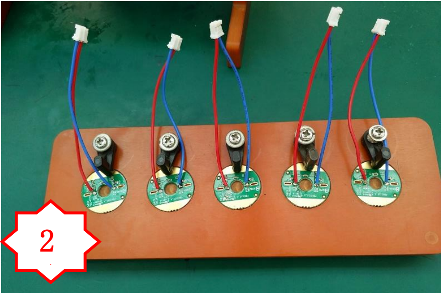
图二，治具辅助焊接
