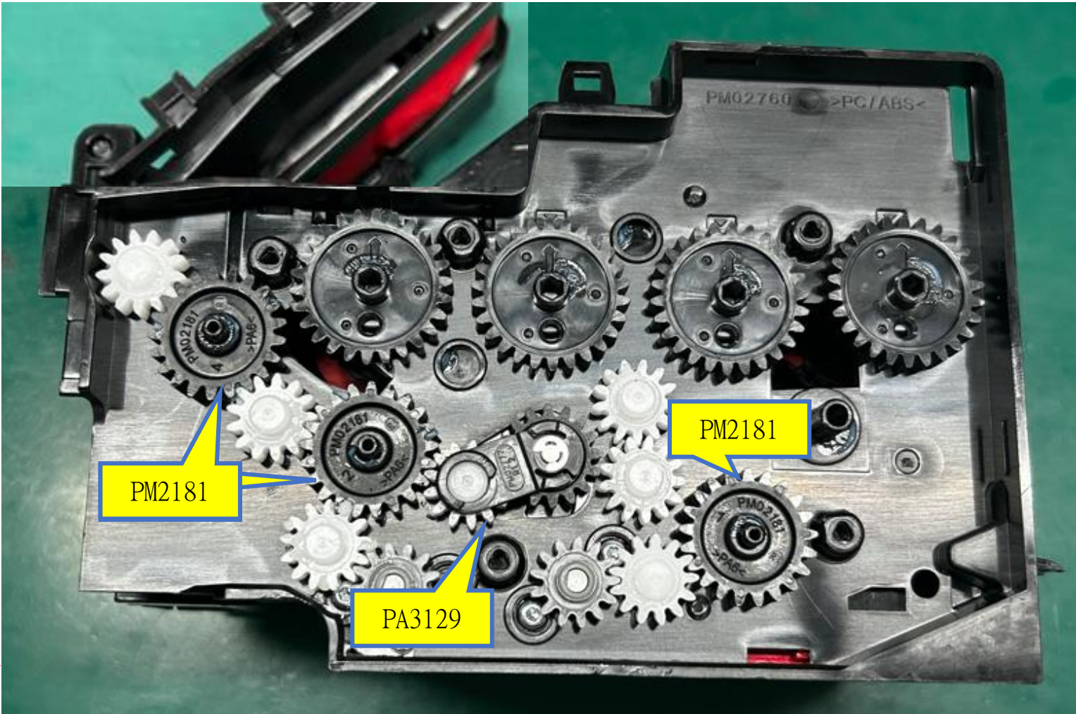
图一，在图示位置装上 3 个 PM2181 和 1 个 PA3129 组件。
