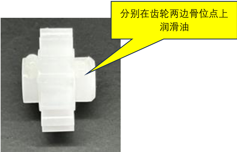
图二, 用点油机在 PM647 两侧的凸台各加大约 0.0071g 油
