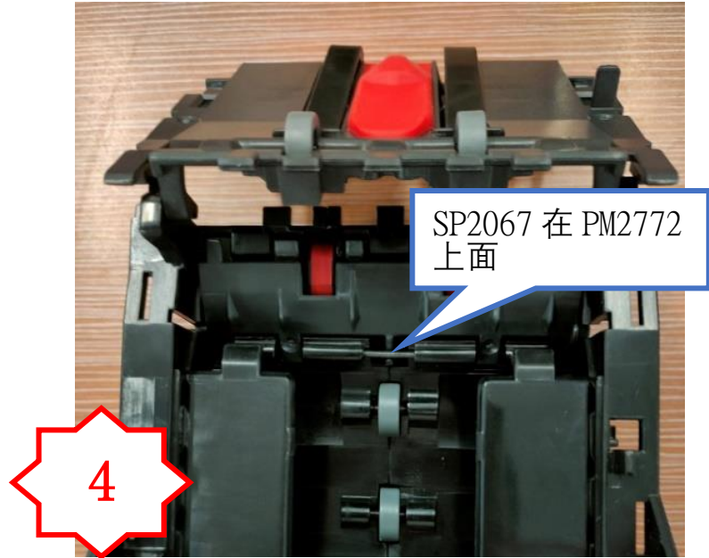
图四，装入后 SP2067 在上面
