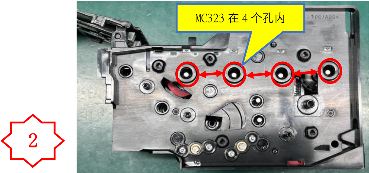
图二, 检查压合后五金轴顶部到胶件圆孔平面深度尺寸: 3.0±0.3mm
