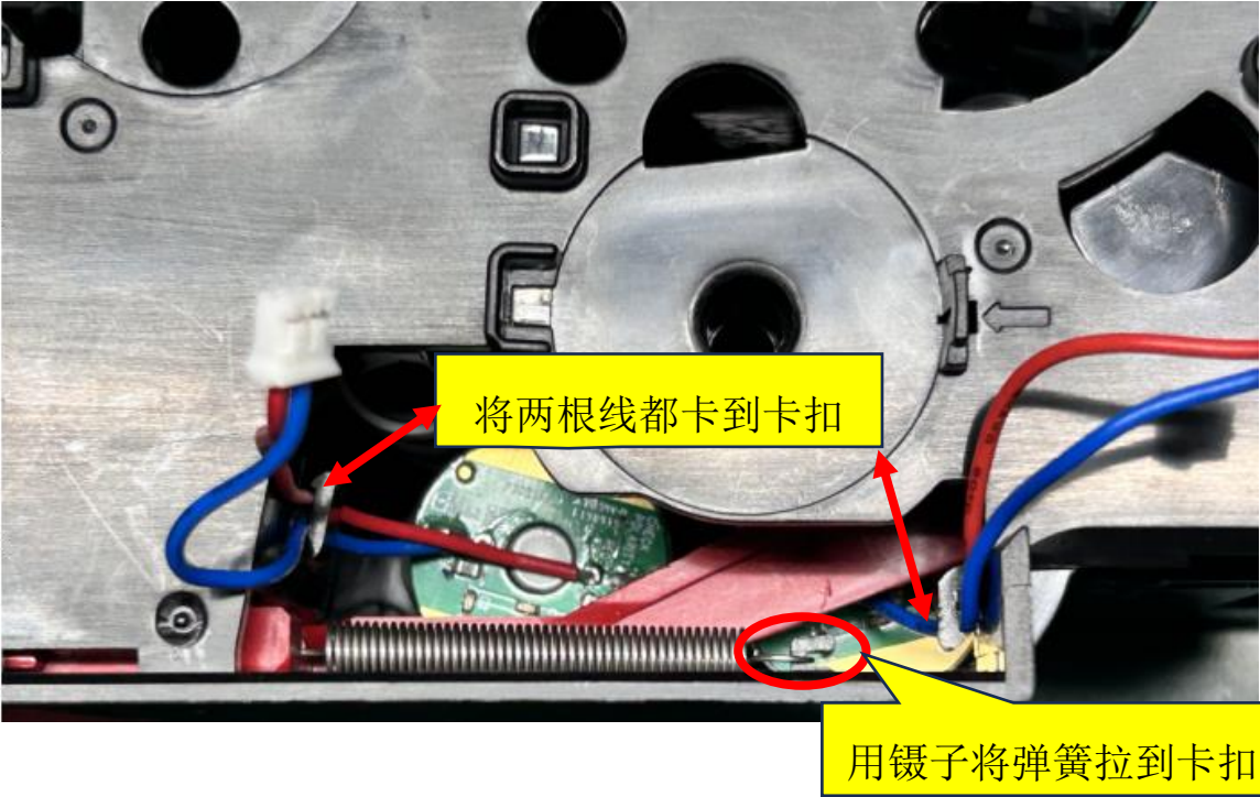
图一，将两根线都卡到卡扣内，用镊子将弹簧拉到卡扣位扣住
