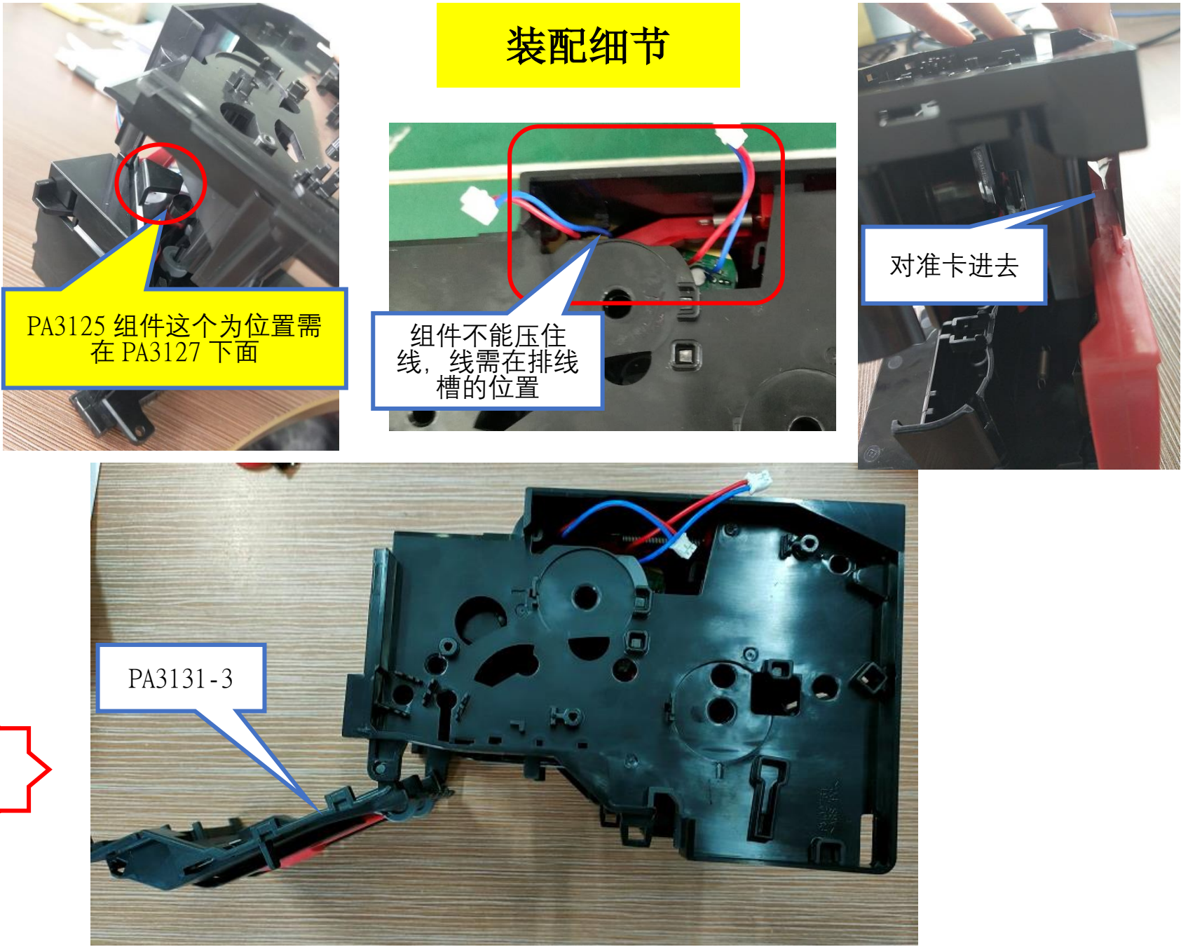
图一，将 PA3125 装入 PA3124-2 组件上，注意装配细节，再将 PA3131-3 装入。
