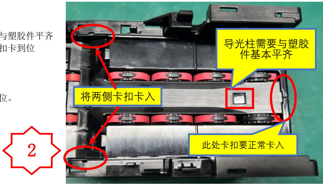
图二，装配到位后，检查两侧卡扣卡到位，导光柱需要与塑胶件平齐。
