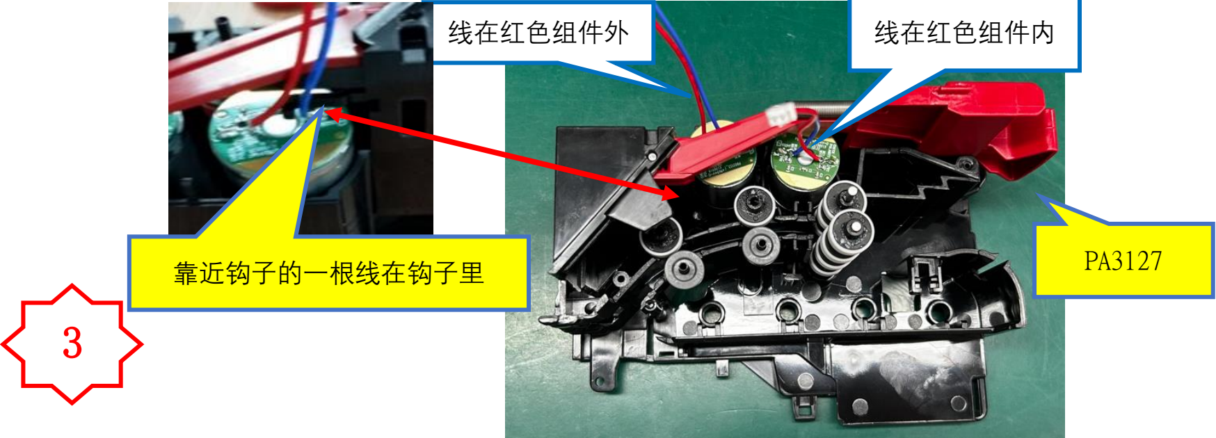
图三, 将 PA3127 装到 PA3124-1 上, 注意红色组件装配位置, 靠近钩子的一根线要在钩子里面。
