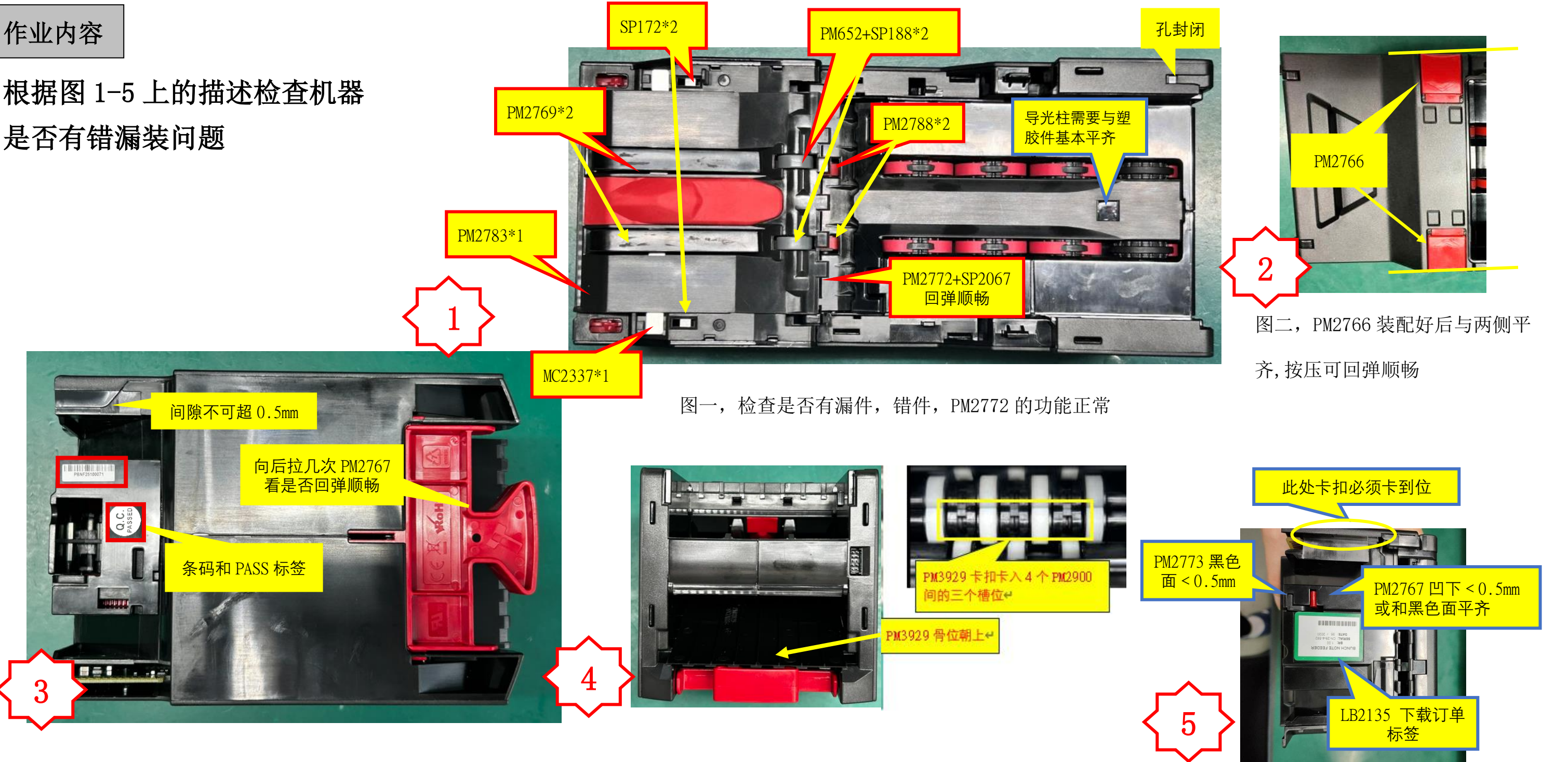
图三，检查 PM2767 功能是否 OK，条码标签和 PASSD（针对打包出货机）是否有贴，侧盖间隙不可超 0.5mm
