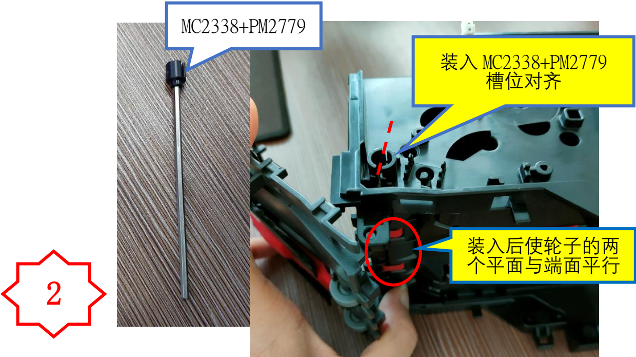
图二, 装入 MC2338+PM2779, 两个轮子的平面需要与平面平齐, PM2779 槽位与 PM2761 上的槽位对齐。
