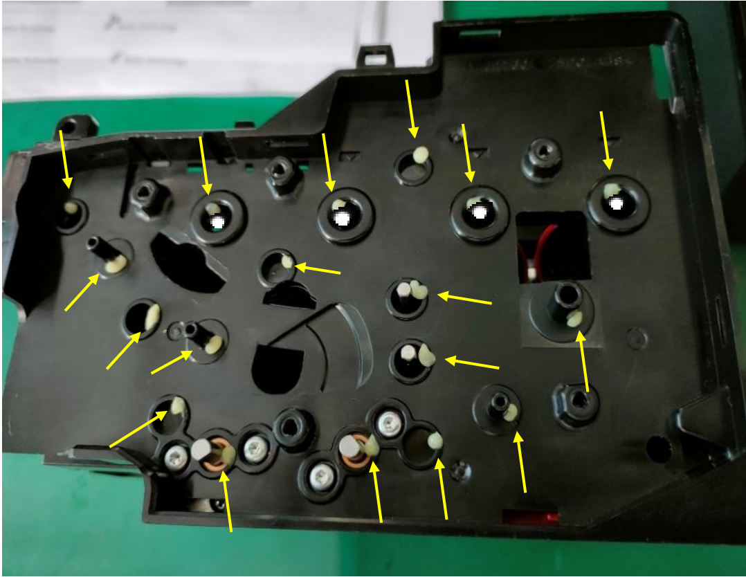
图一，用点油机在 18 处各加大约 0.0071g NYE368F 油
