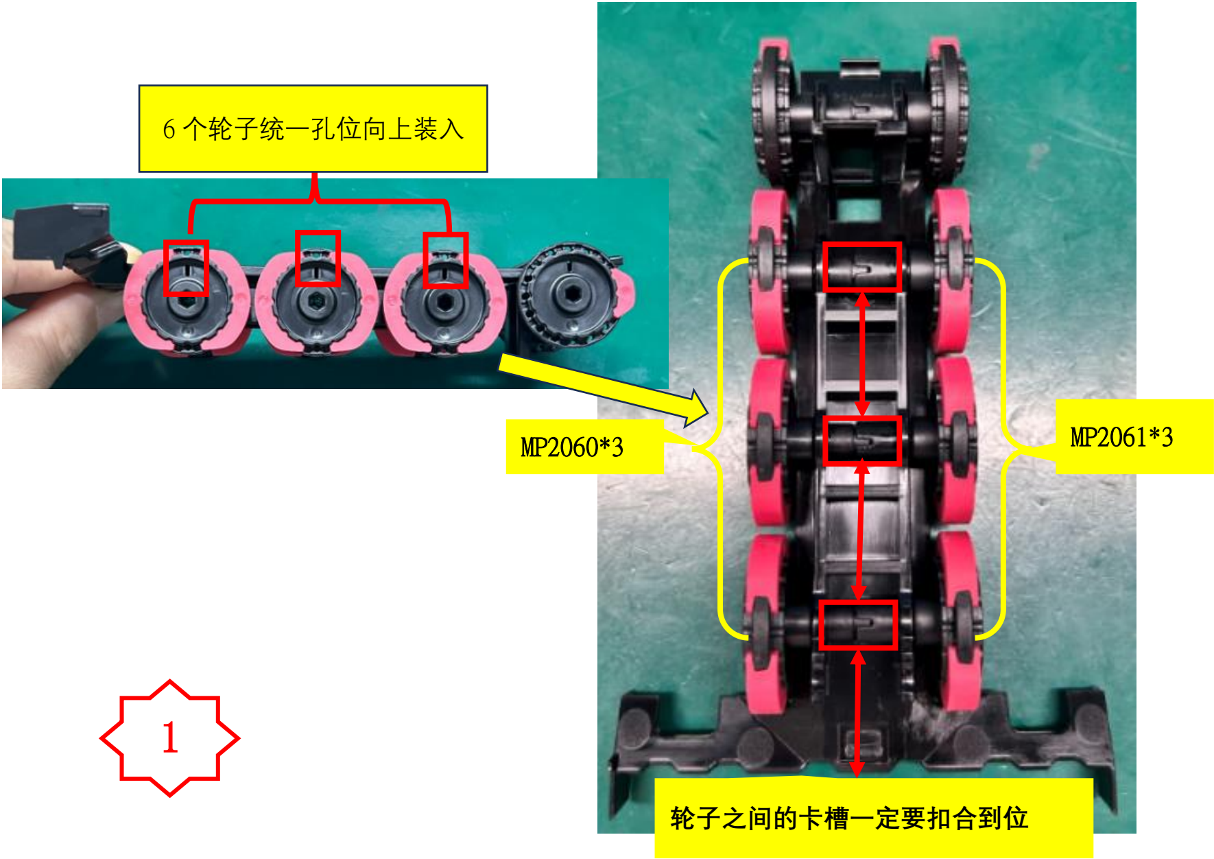
图一，将 6 个轮子长孔位朝上统一装进 PM2771 组件, 注意装配位置及方向，轮子之间的卡槽一定要扣合到位。
