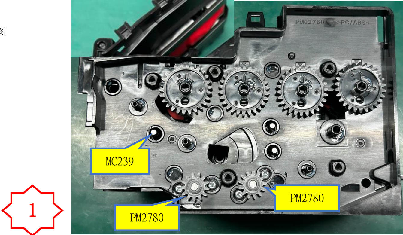
图一，在 PA3122-4 的马达轴上装入两个 PM2780，注意平面朝下方向装入，再装入 1 根 MC239 如图所示位置。
