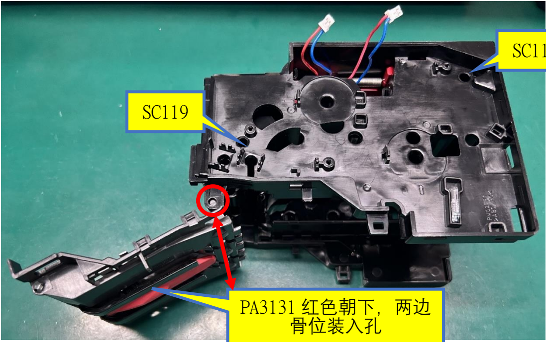
图一，确认 PA3131 红色朝下将两边骨位装到 PA3124-3 两边孔，再打 2 颗 SC119
