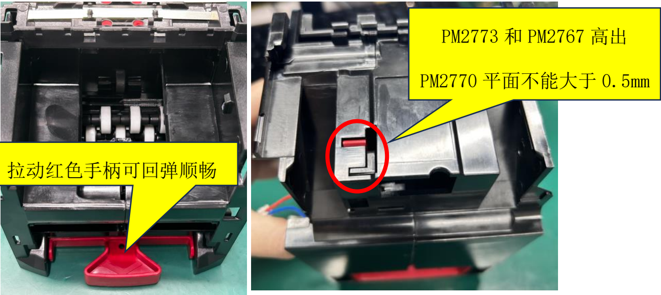
图二，检查拉动红色手柄可以回弹顺畅，PM2773 和 PM2767 高出 PM2770 平面不能大于 0.5mm
