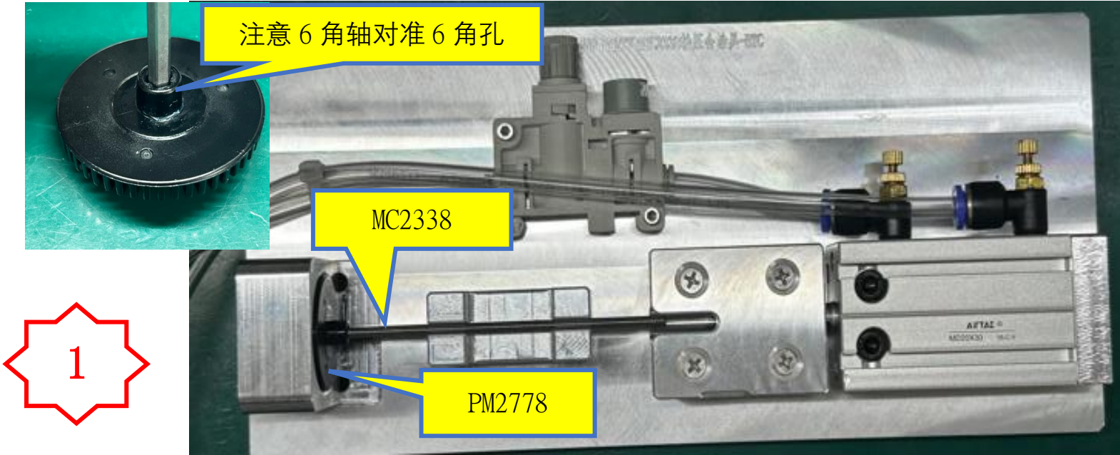
图一，先将 MC2338 轴预装入 PM2778，注意 6 角轴对准 6 角孔，确认装到位后再进行压合。
