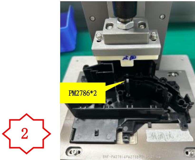
图二，将 2 个 PM2786 预装入 PA3125-1 上的 PM2761 中，再用治具压合。
