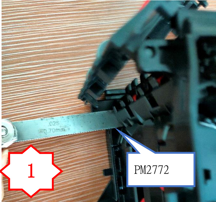
图一，在 PM2772 底部塞入一根 0.7mm 的塞尺
