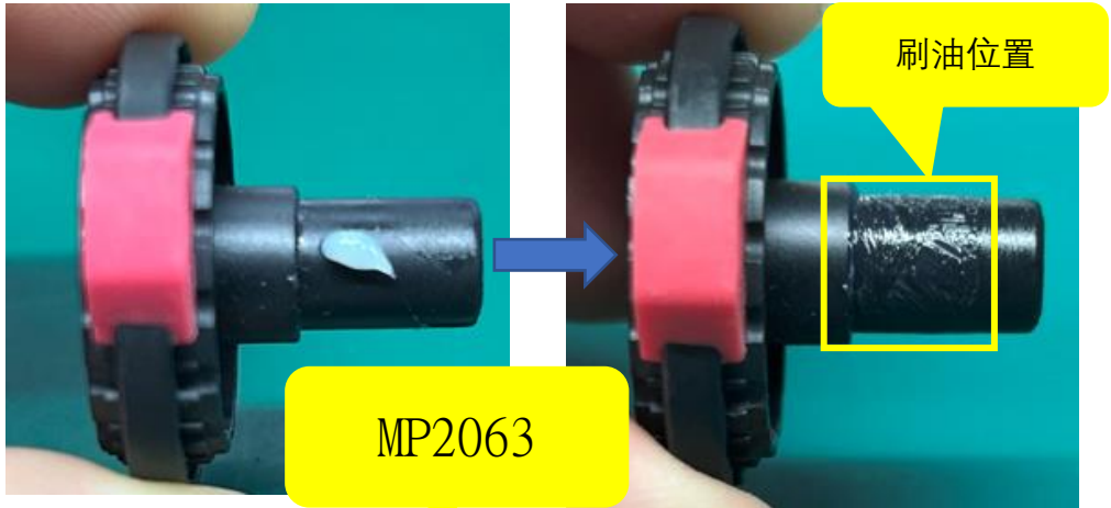
图二，用点油机在 MP2063 加大约 0.0071g NYE368 油，然后用毛刷将油均匀刷在柱子上。
