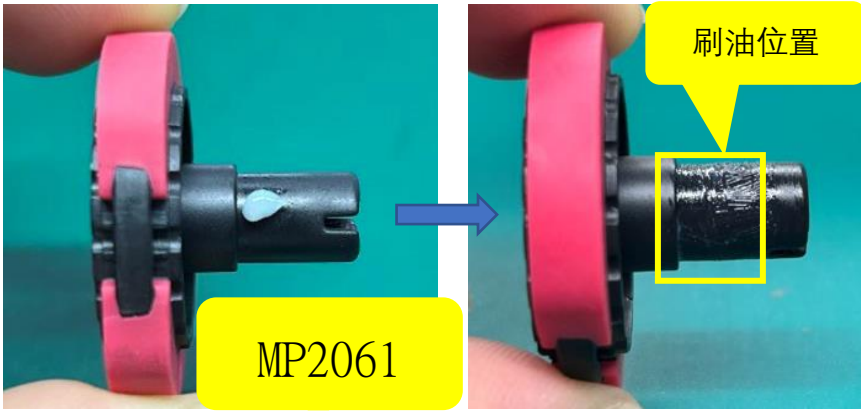
图二，用点油机在 MP2061 加大约 0.0071g NYE368 油，然后用毛刷将油均匀刷在柱子上。
