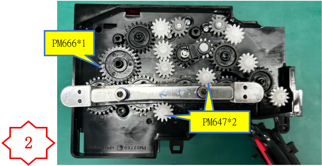
图二，将 1 个 PM666 和 2 个 PM647 孔朝下装到对应位置，装配完成后再取出治具。
