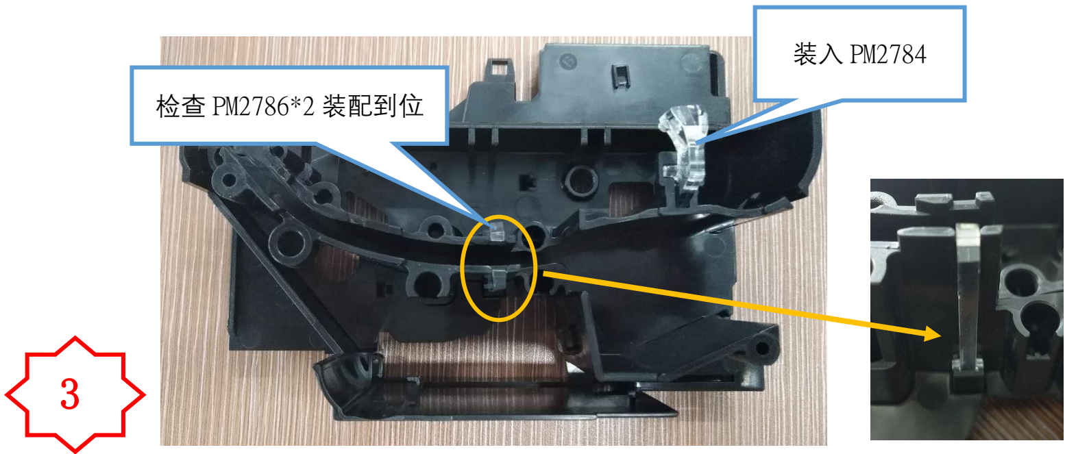
图二，检查 PM2786*2 装配到位，然后装入一个 PM2784。
