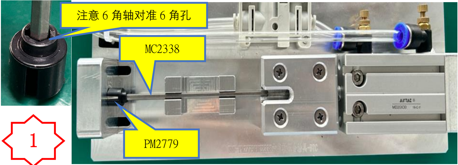
图一，先将 MC2338 轴预装入 PM2779，注意 6 角轴对准 6 角孔，确认装到位后再进行压合。
