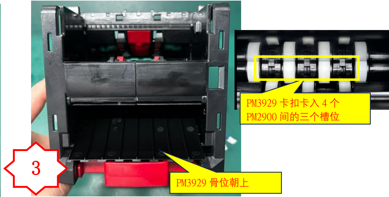
图三，在 PM2900 四个轮子间的 3 个槽位卡入 PM3929, 注意 PM3929 的方向骨位朝上，装配到位后活动顺畅。
