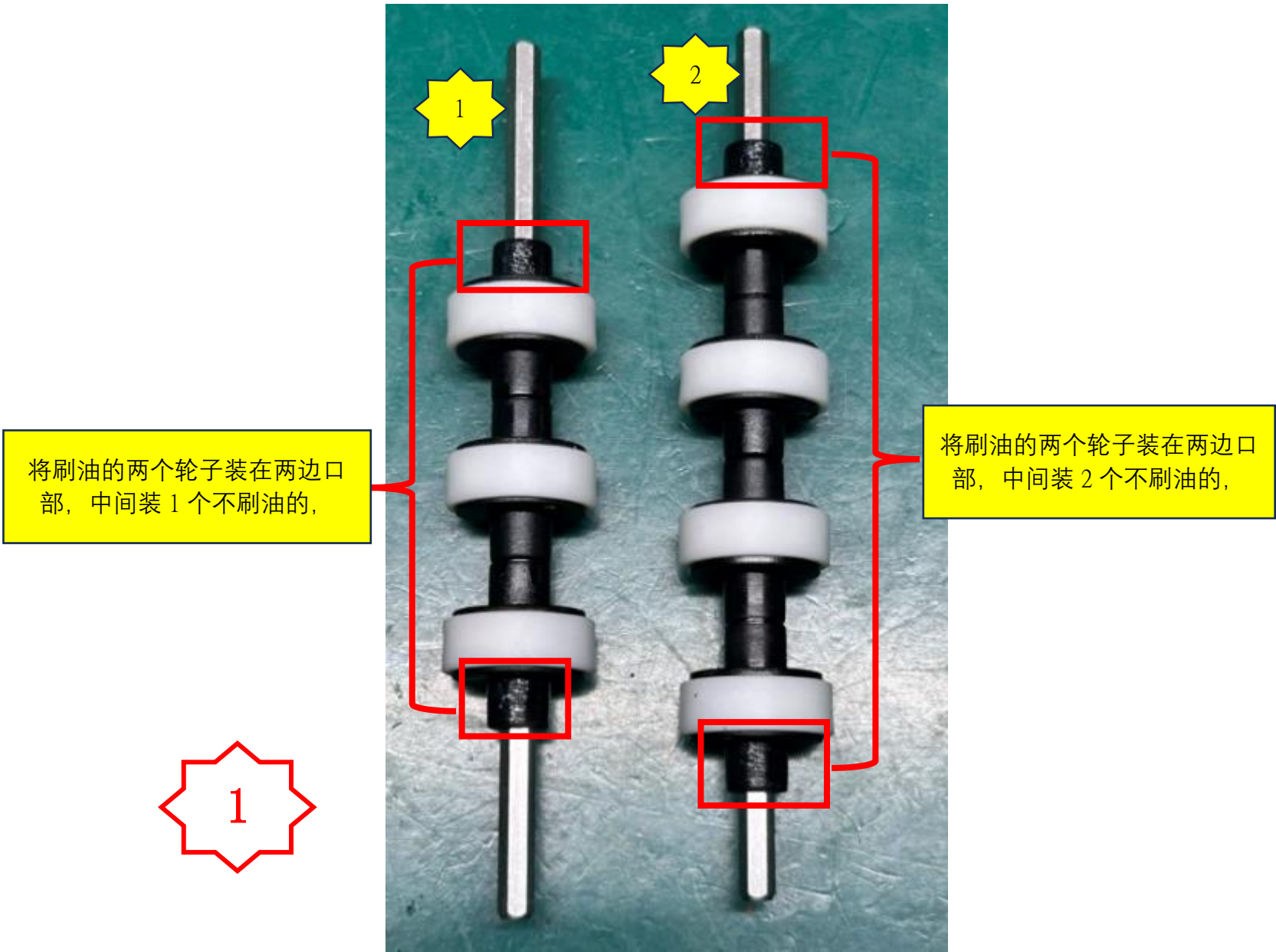
图一, 在 MC239 五金轴①上装上 1 个 PM2900, 再将刷了单边油的 PM2900 分别装在轴的两端口部位置, 在 MC239 五金轴②上装上 2 个 PM2900, 再将刷了单边油的 PM2900 分别装在轴的两端口部位置.
