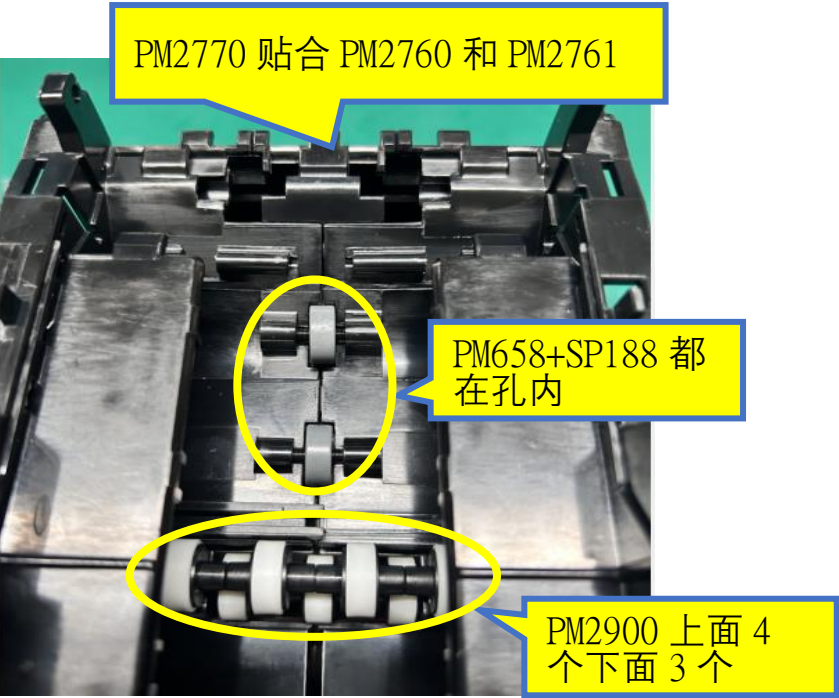
图二，锁螺丝后检查是否有错漏问题
