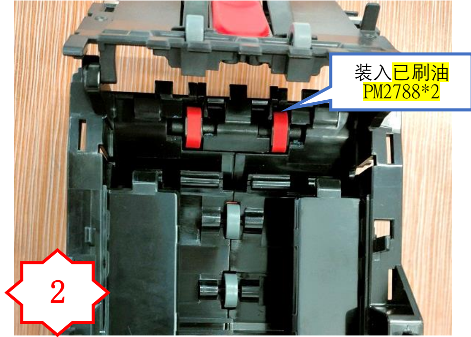
图二，装入两个 PM2788
