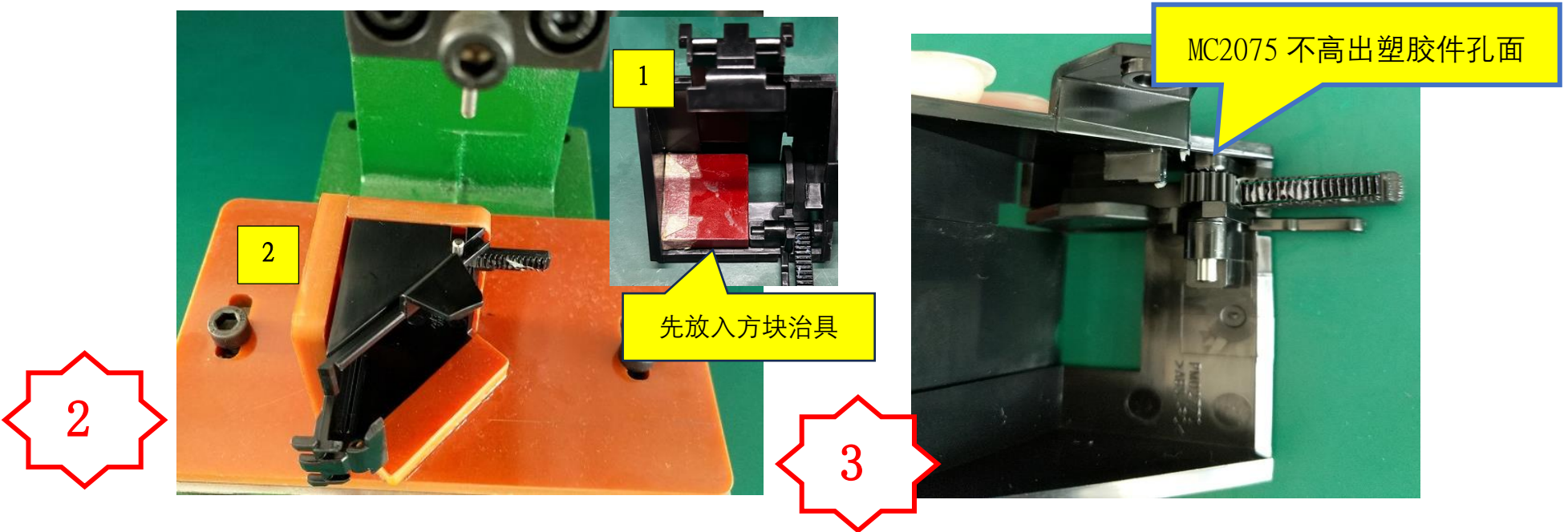
图二, 将组件先装入方块支撑治具, 再放到定位治具上进行压合 MC2075 轴。
