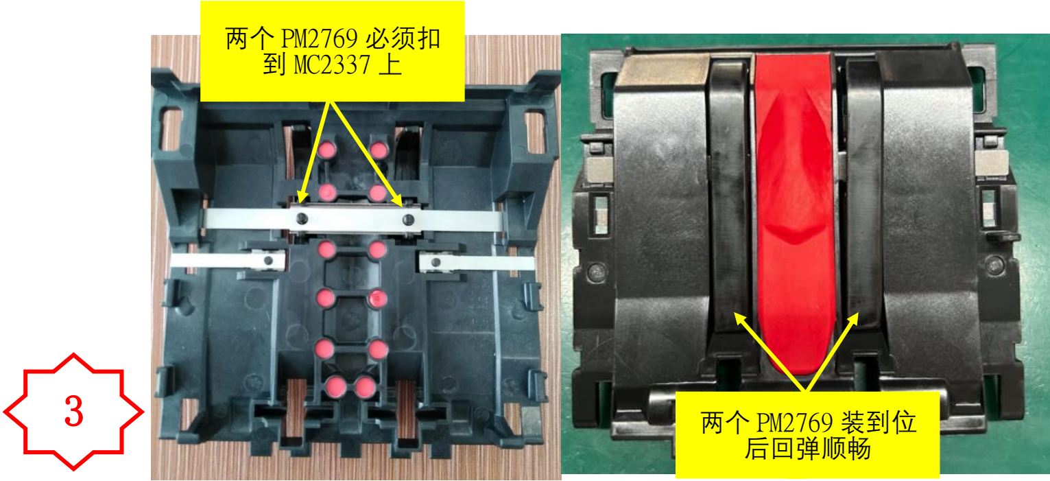
图三, 装入两个 PM2769, 注意卡扣需扣到 MC2337 上, 检查两个 PM2769 装到位后回弹顺畅。
